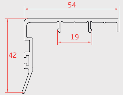
SÜRME ALIN KAPAMA ( Interlocking Profile )
