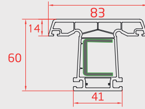
KAPI İÇİ ORTA KAYIT (Door Sash Mullion Profile)
