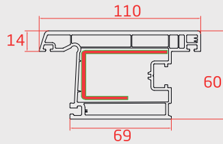
DIŞA AÇILIR KAPI (Outward Opening Door Sash Profile)
