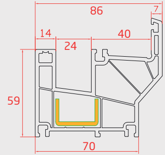
SÜRME TEKLİ KASA ( Fixed Frame Slider )
