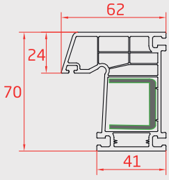
KASA (Frame Profile)
