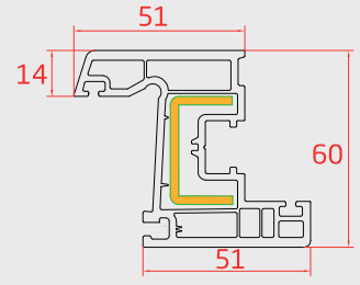
KANAT (Sash Profile)
