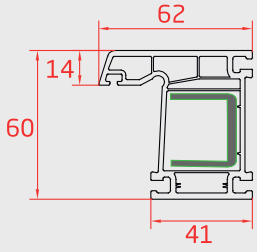
KASA (Frame Profile)
