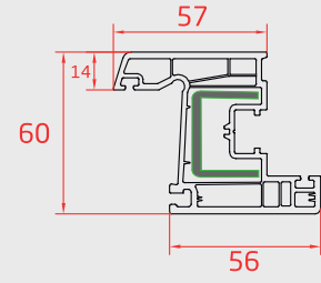
KANAT (Sash Profile)
