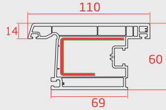
DIŞA AÇILIR KAPI (Outward Opening Door Sash Profile)
