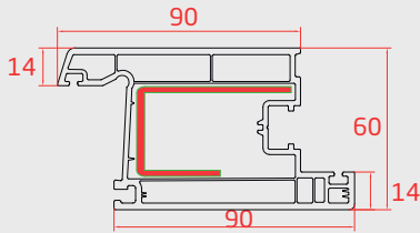
İÇE AÇILIR KAPI (Door Sash Profile)
