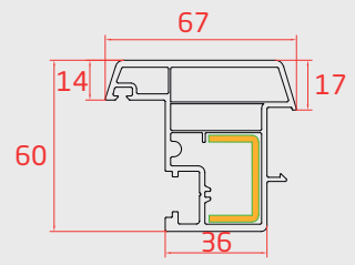
HAREKETLİ ORTA KAYIT (Overhung Profile)
