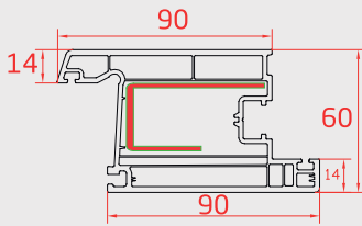
İÇE AÇILIR KAPI (Door Sash Profile)
