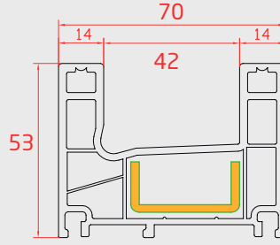
SÜRME KASA ( Sliding Frame Profile )
