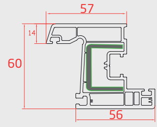
KANAT (Sash Profile)
