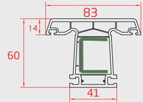
KAPI İÇİ ORTA KAYIT (Door Sash Mullion Profile)
