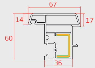
HAREKETLİ ORTA KAYIT (Overhung Profile)
