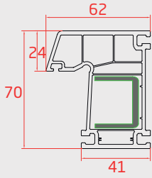
KASA (Frame Profile)
