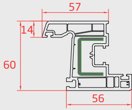
KANAT (Sash Profile)
