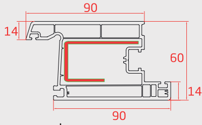
İÇE AÇILIR KAPI (Door Sash Profile)
