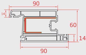
İÇE AÇILIR KAPI (Door Sash Profile)
