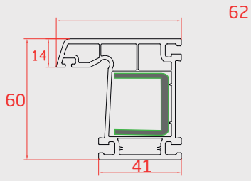
KASA (Frame Profile)
