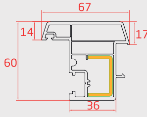
HAREKETLİ ORTA KAYIT (Overhung Profile)
