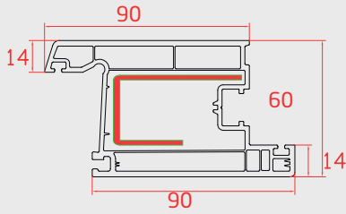
İÇE AÇILIR KAPI (Door Sash Profile)
